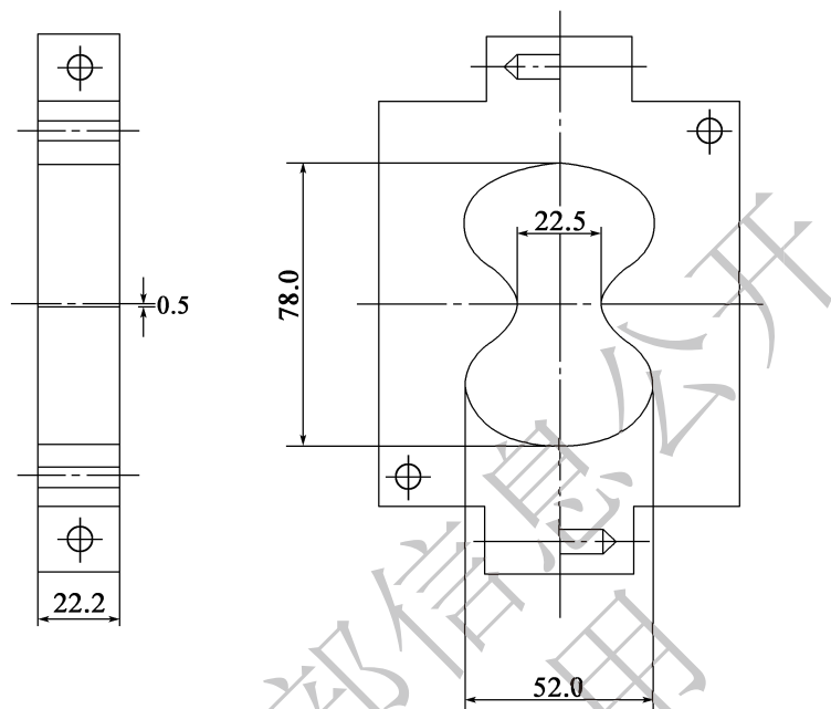
图 B.3.2 “8”字形金属模具（尺寸单位：mm）
