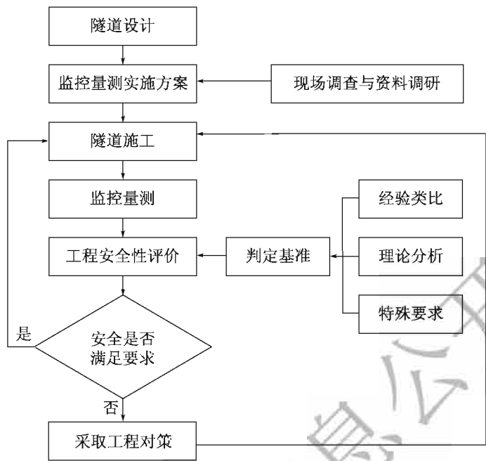
图 18.6.2 信息反馈程序框图
