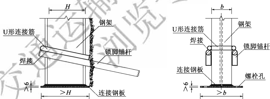
图 9-5 锁脚锚杆安装说明图 (尺寸单位: mm)
