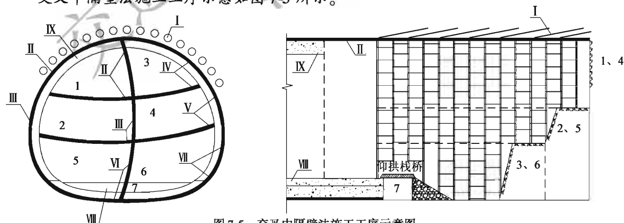
图 7-5 交叉中隔壁法施工工序示意图
