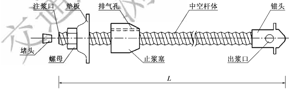
图 9-3 中空锚杆说明图
