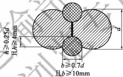
图 9-8 焊缝要求
