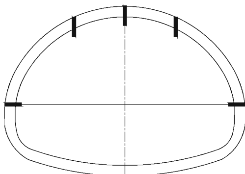
图 18-1 全断面法测点布置
