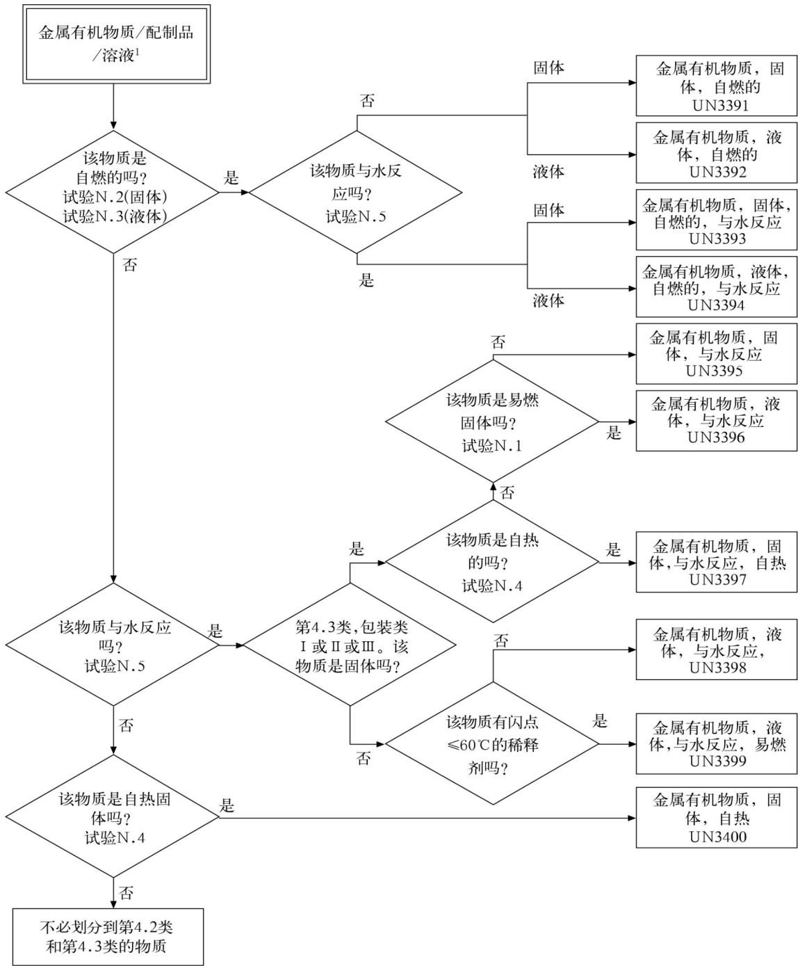
金属有机物质的流程图 1,2
