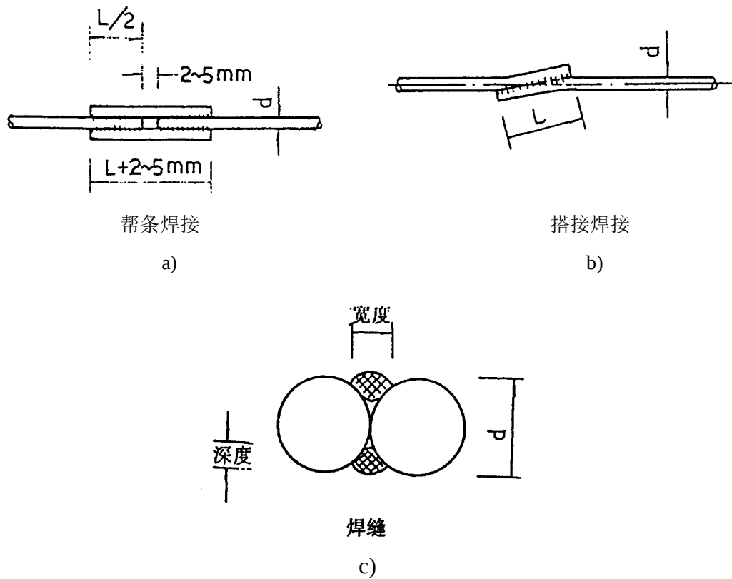
图403-1 电弧焊接
