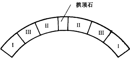
图413-7 拱圈砌筑
