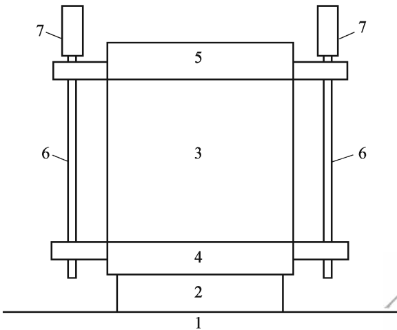
图 T 0713-1 变形量测装置
