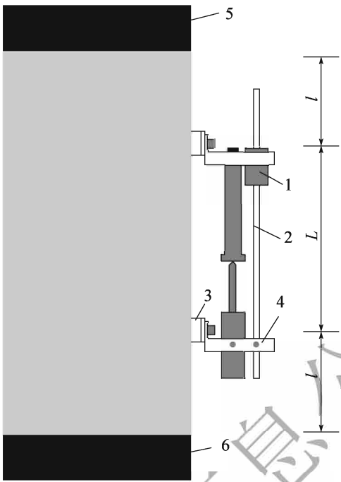
图 T 0738-2 位移传感器安装示意图
