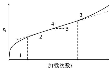
图 T 0745-7 累计应变-加载次数曲线
