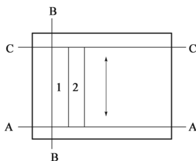
图 T 0703-6 切割棱柱体试件的顺序
