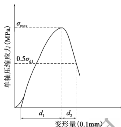
图 T 0774-1 单轴压缩试验强度-变形量曲线
