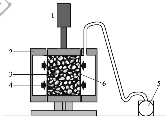
图 T 0745-2 B 型三轴重复压缩试验装置 1-动力制动器;2-压力室;3-试件;4-围压;5-真空泵; 6-轮胎内胎
