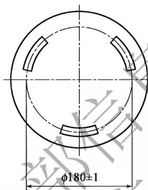
图 T 0760-5 摩擦测头(尺寸单位:mm)
