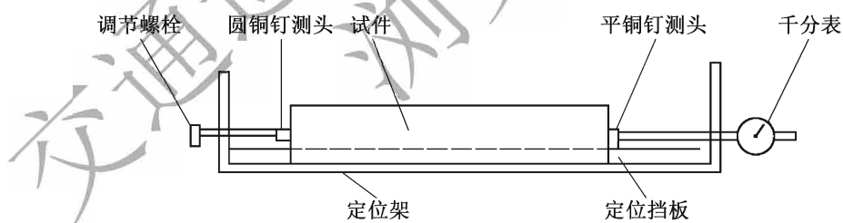
图 T 0720-1 沥青混合料收缩试验仪
