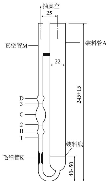
图 T 0620-3 CMVV 式真空减压毛细管黏度计 (尺寸单位:mm)
