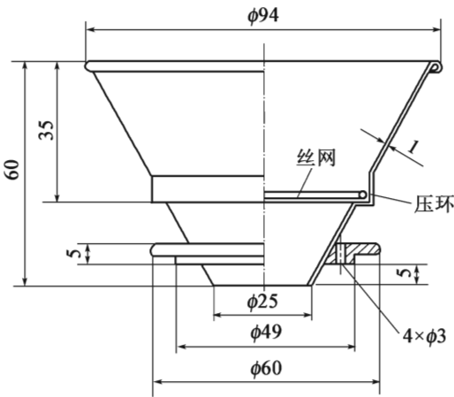
图 T 0623-5 过滤漏斗(尺寸单位:mm)
