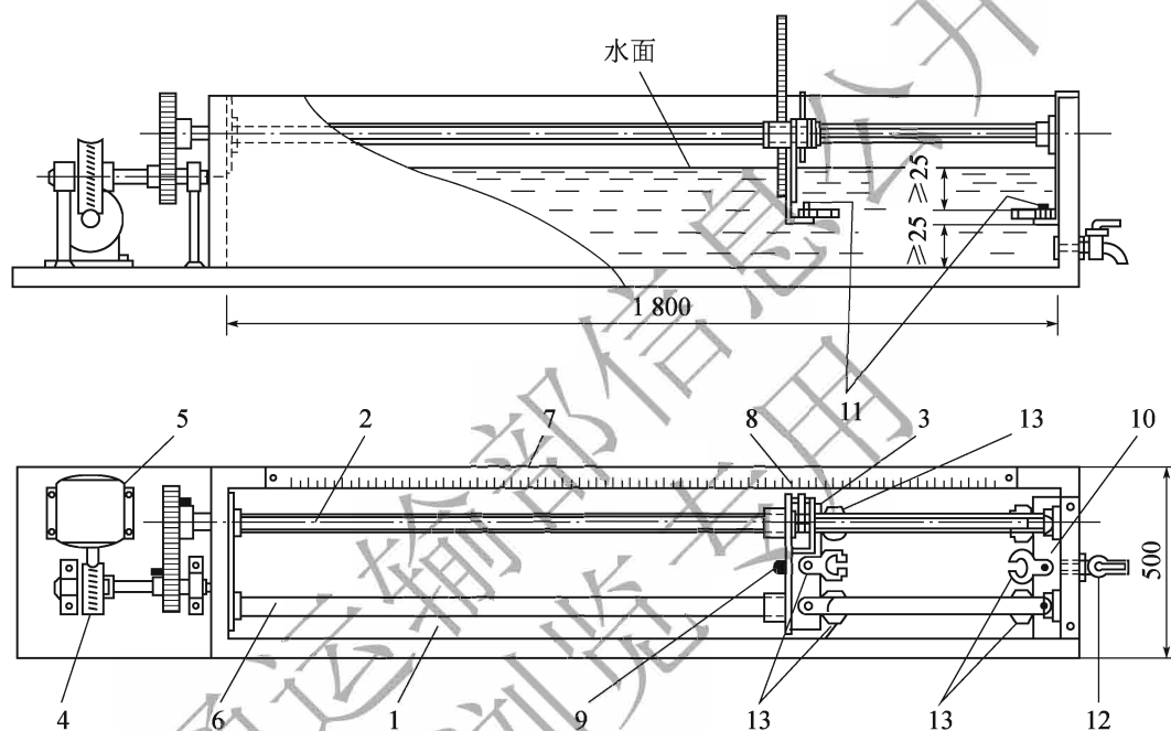
图 T 0605-1 典型延度仪(尺寸单位:mm)
