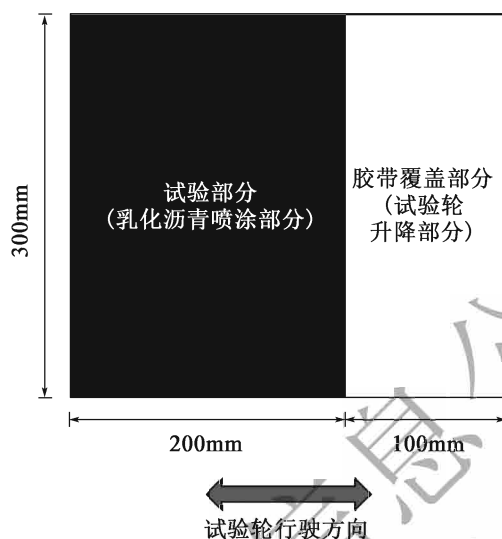
图 T 0672-1 试验轮下降前涂布基板胶带遮挡示意图
