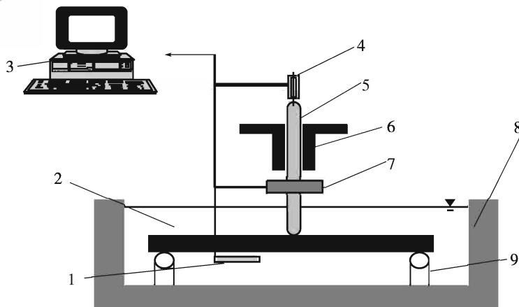
图 T 0627-1 弯曲梁流变仪
