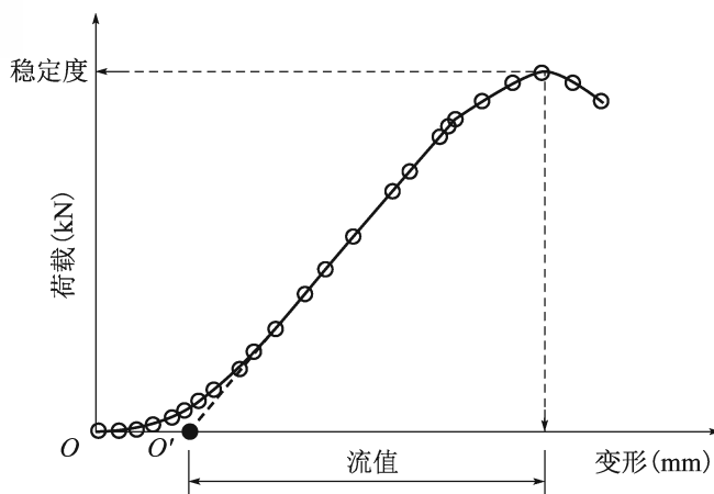
图 T 0709-2 稳定度-变形量曲线原点修正示意图
