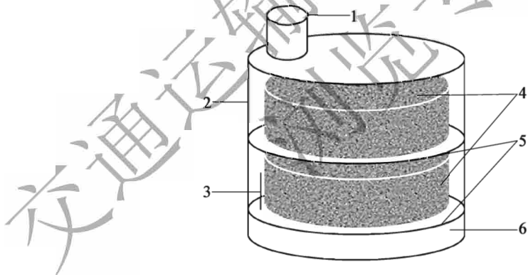
图 T 0749-1 压力室
