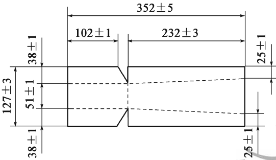
图 T 0667-4 锡防护罩(尺寸单位:mm)
