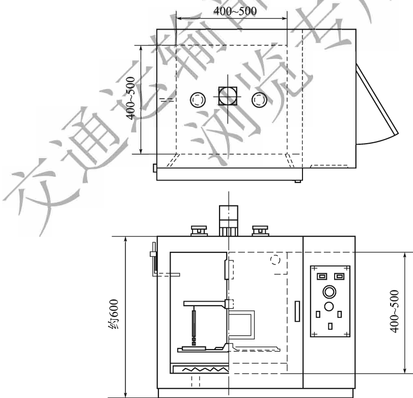
图 T 0609-1 薄膜烘箱(尺寸单位:mm)
