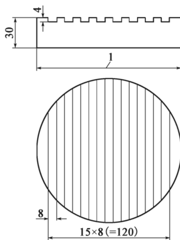
图 T 0772-3 扩展件表面刻槽示意图 (尺寸单位: mm) 1-扩展件的直径与试件直径匹配
