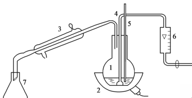
图 T 0726-1 蒸馏装置
