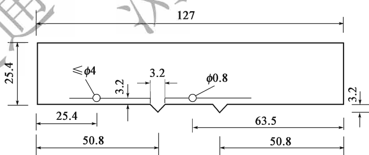
图 T 0633-3 量规(尺寸单位:mm)
