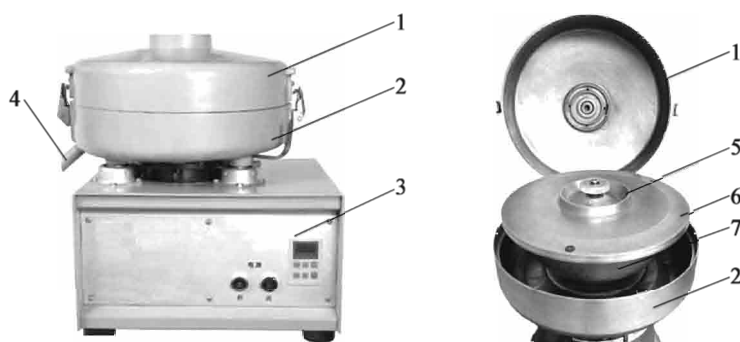
图 T 0722-4 离心抽提仪
