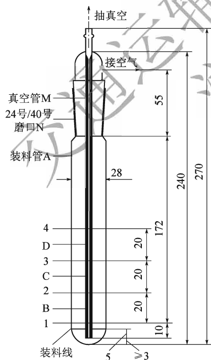
图 T 0620-2 MKVV 式真空减压毛细管黏度计 (尺寸单位:mm)
