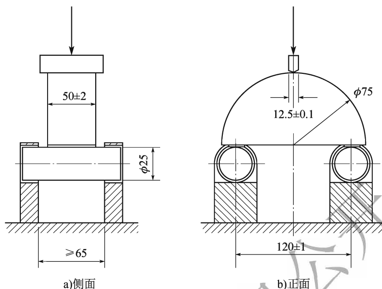
图 T 0744-2 半圆弯曲加载图示及其尺寸要求(尺寸单位:mm)
