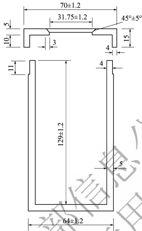
图 T 0638-1 盛样瓶(尺寸单位:mm)
