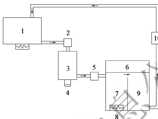
图 T 0722-3 筛塔式自动抽提仪
