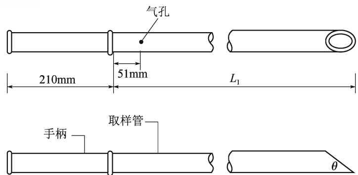
图 T 0601-7 带气孔的取样管
