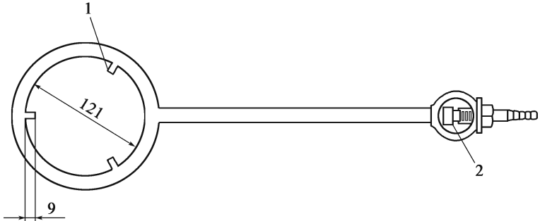
图 T 0667-3 环形燃烧器(尺寸单位:mm)
