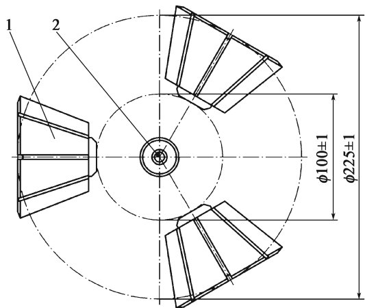
图 T 0760-2 磨光盘(尺寸单位:mm)
