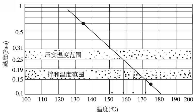
图 T 0625-3 由沥青结合料的黏温曲线确定施工温度
