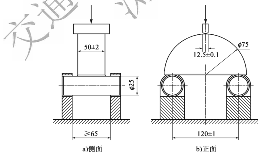
图 T 0747-1 半圆弯曲加载图示及其尺寸要求(尺寸单位:mm)
