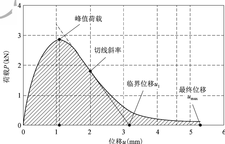
图 T 0744-6 记录的荷载 P 与位移 u 曲线
