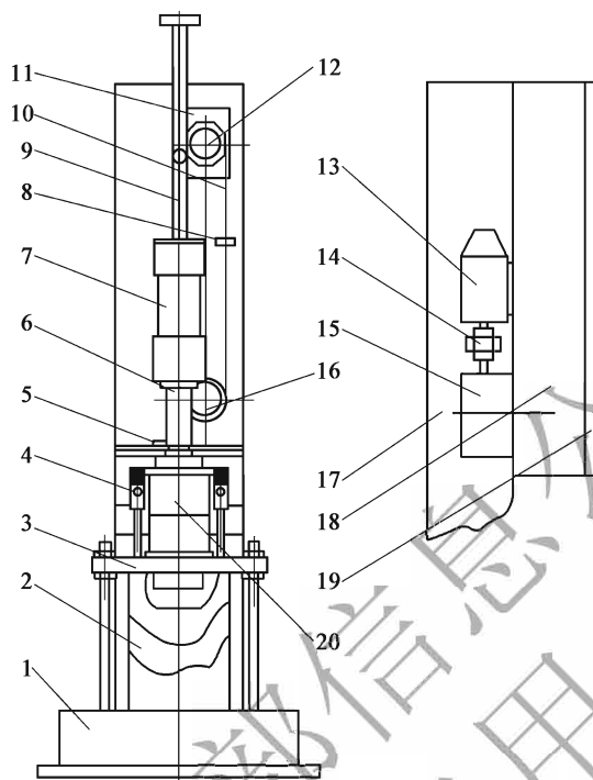
图 T 0702-1 沥青混合料马歇尔击实仪
