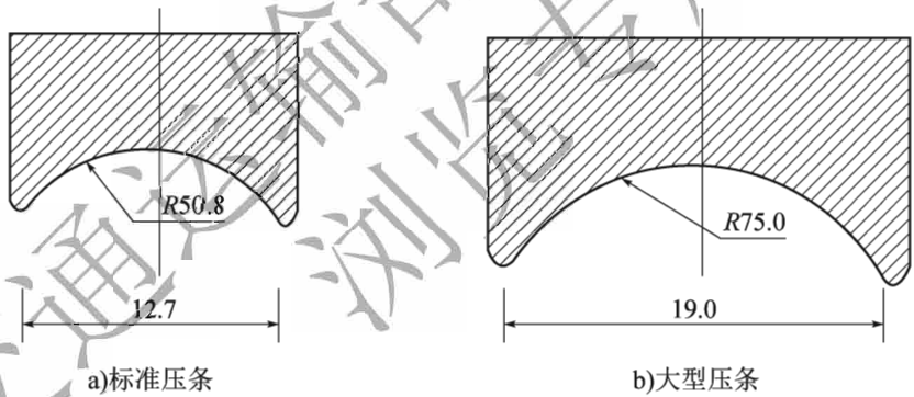
图 T 0716-2 压条(尺寸单位:mm)
