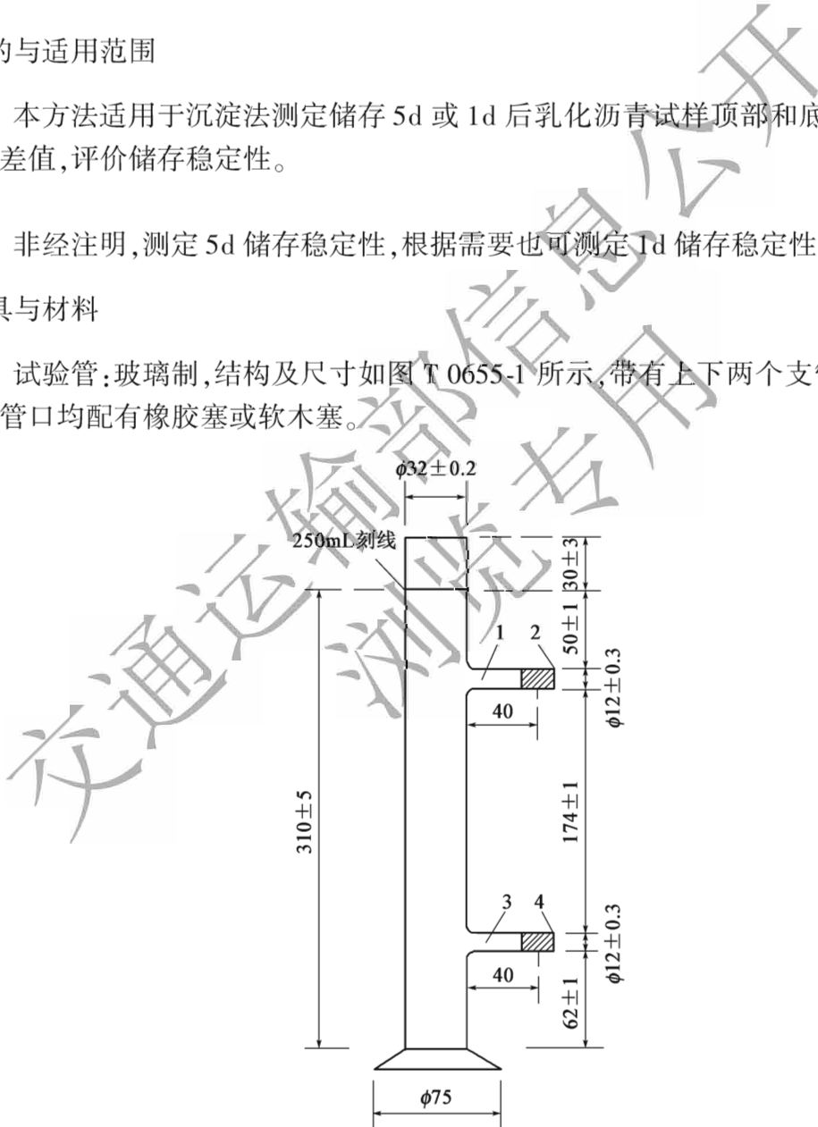
图 T 0655-1 试验管(尺寸单位:mm)
