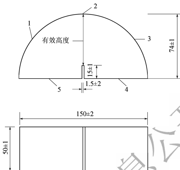
图 T 0744-4 试件切缝示意图及尺寸要求 (尺寸单位:mm)
