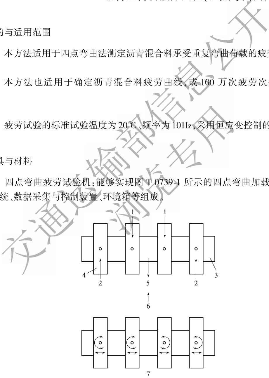
图 T 0739-1 四点弯曲加载图示
