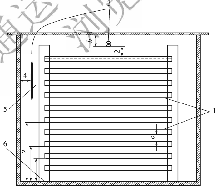
图 T 0630-2 压力容器 (PAV) 内部结构
