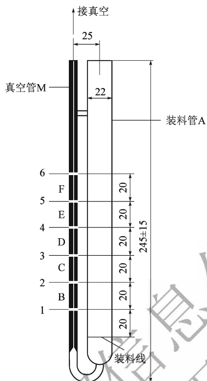
图 T 0620-1 AIVV 式真空减压毛细管黏度计(尺寸单位:mm)
