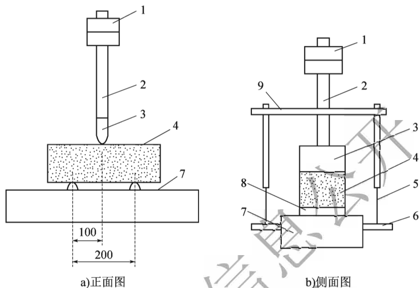
图 T 0715-1 加载装置(尺寸单位:mm)
