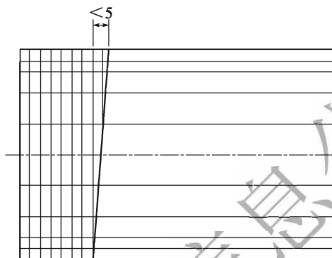
图 T 0772-4 试件层间界面倾斜度(尺寸单位:mm)
