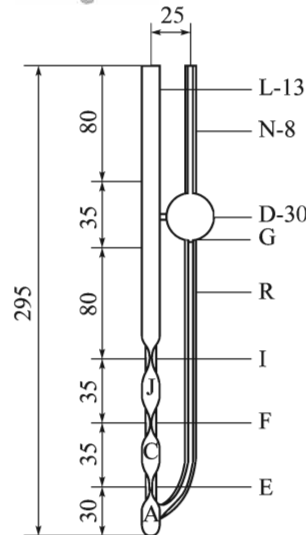
图 T 0619-1 坎芬式逆流毛细管黏度计(尺寸单位:mm)
