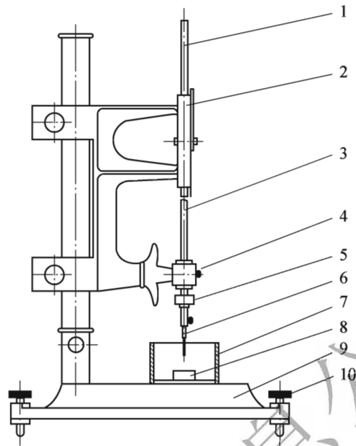
图 T 0604-1 针入度仪
