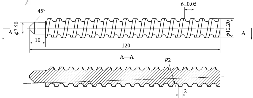
图 T 0638-2 右旋螺纹的螺杆(尺寸单位:mm)
