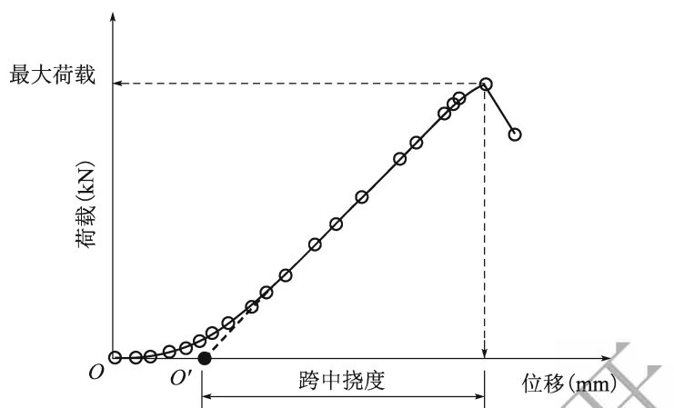
图 T 0715-2 弯曲试验荷载-跨中挠度曲线
