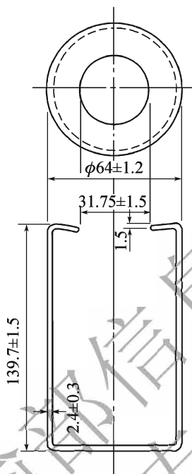
图 T 0610-3 盛样瓶 (尺寸单位: mm)
