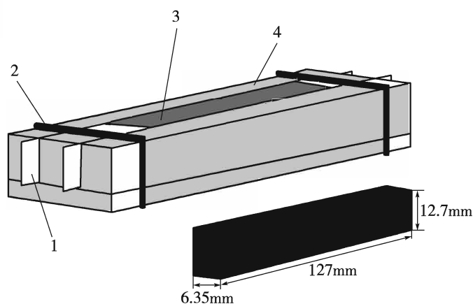
图 T 0627-5 试件成型示意图(铝制试模) 1-塑料片;2-O 形橡胶圈;3-沥青试件;4-铝制试模
