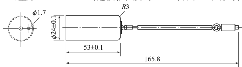
图 T 0639-1 转子示意图及尺寸(尺寸单位:mm)
