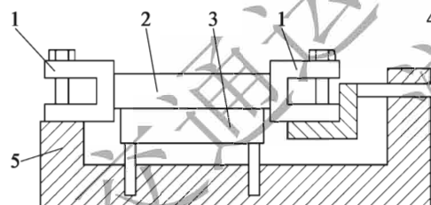
图 T 0748-3 试件安装台
