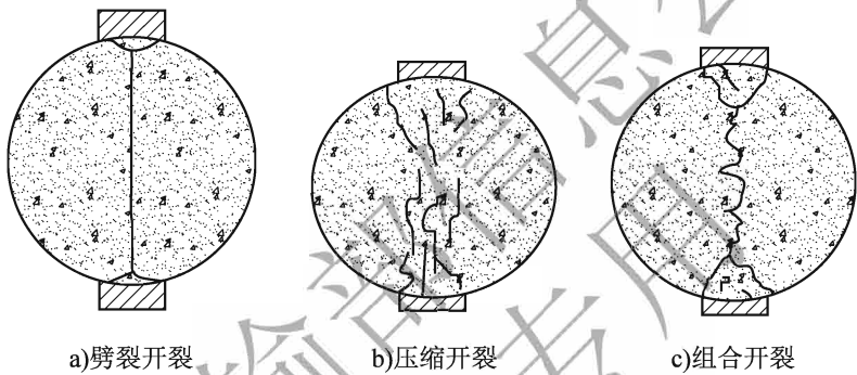
图 T 0716-3 试件破坏形式示意图
