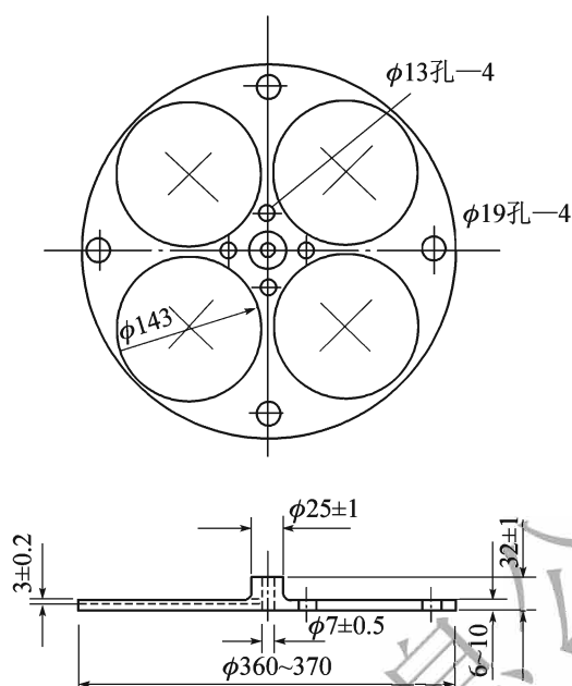
图 T 0609-2 圆盘架(尺寸单位:mm)
