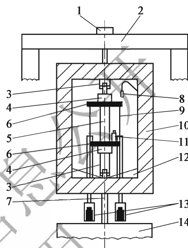
图 T 0748-2 位移传感器外置式低温约束应力试验仪 1-荷载传感器;2-加载架;3-旋转夹具;4-夹头;5-试件;6-下加载板;7-加载杆;8-温度传感器;9-钢筋棒;10-环境箱;11-内置温度传感器的混合料小梁;12-风扇;13-位移传感器;14-步进电机
