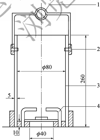
图 T 0601-2 底部进样取样器 (尺寸单位:mm)
