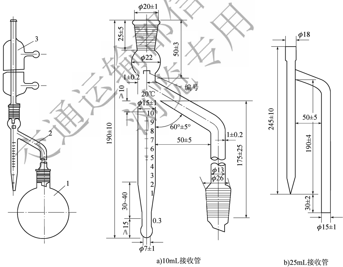
图 T 0612-1 含水率测定仪 1-烧瓶;2-水分接收器;3-冷凝管
