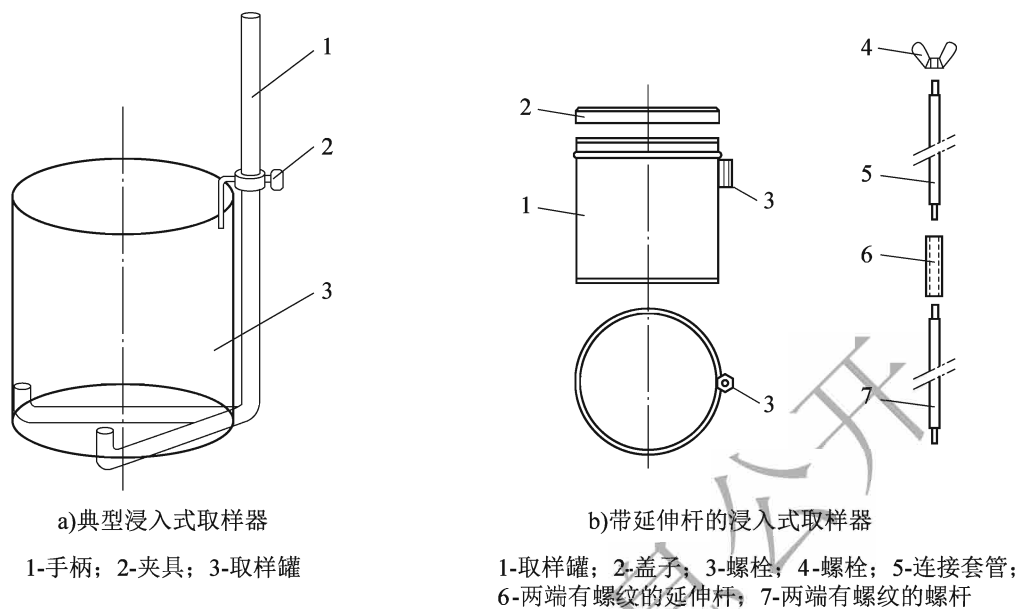
图 T 0601-3 带手柄(延伸杆)的取样器
