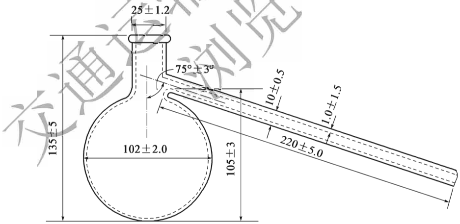
图 T 0632-2 蒸馏烧瓶(尺寸单位:mm)
