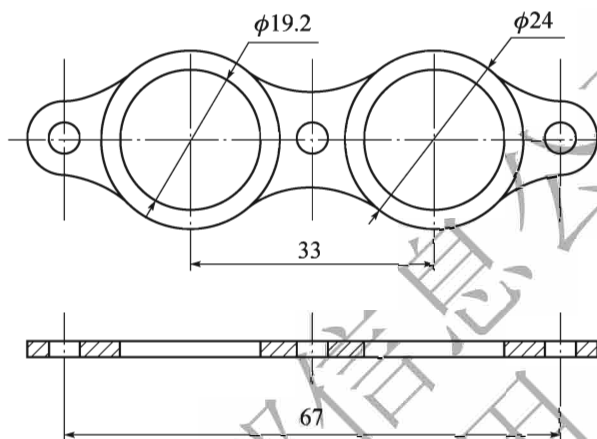
图 T 0606-4 中层板 (尺寸单位: mm)
