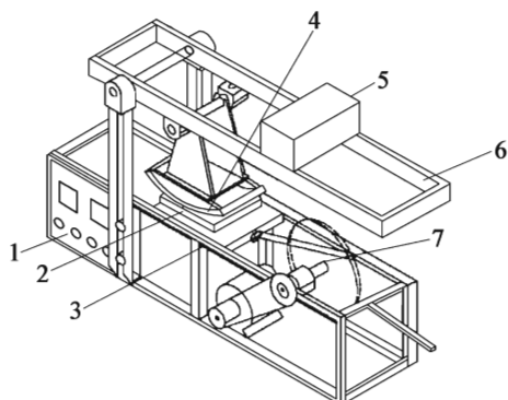
图 T 0703-1 配重式轮碾成型机
