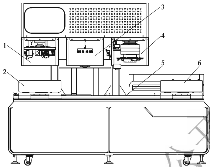
图 T 0760-1 沥青混合料加速磨光试验仪(整体式)
