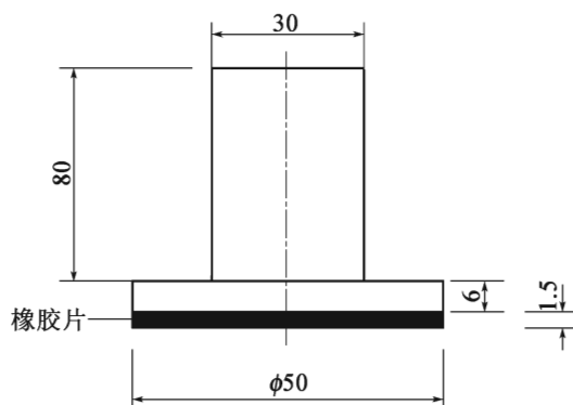
图 T 0731-2 推平板(尺寸单位:mm)
