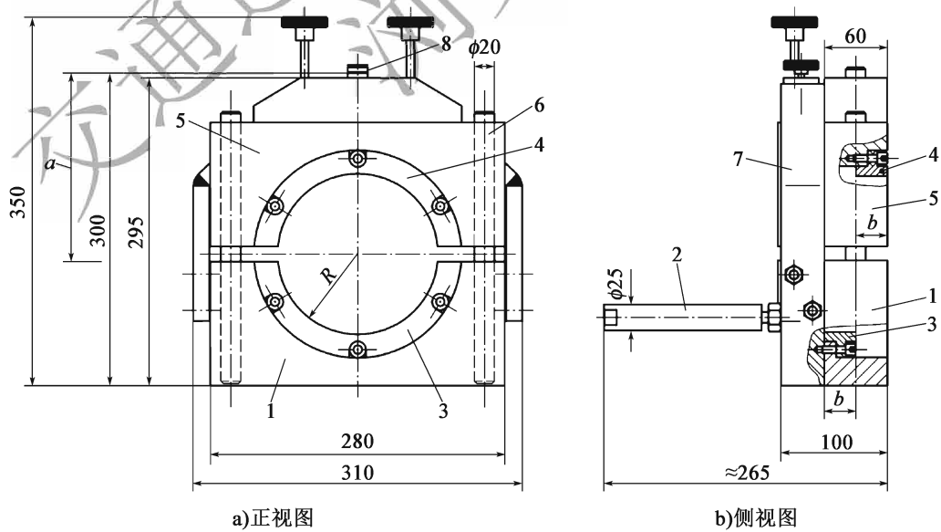
图 T 0772-1 剪切仪(尺寸单位:mm)
