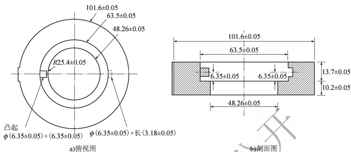
图 T 0649-2 试模(尺寸单位:mm)
