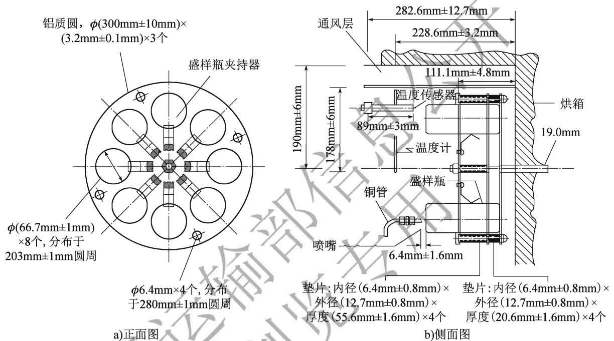
图 T 0610-2 环形金属架
