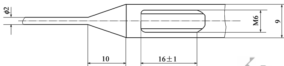
图 T 0613-4 金属锥(尺寸单位:mm)
