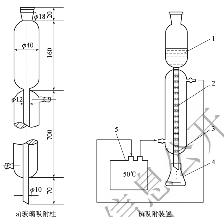
图 T 0618-2 玻璃吸附柱及吸附装置(尺寸单位:mm) 1-冲洗剂;2-氧化铝;3-脱脂棉;4-磨口锥形瓶;5-恒温水槽
