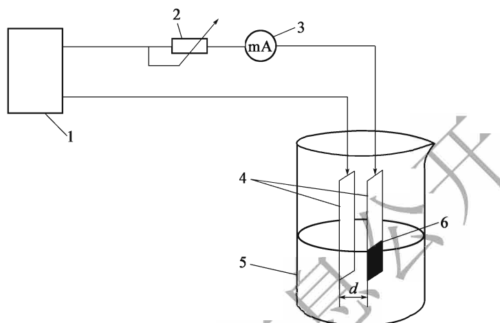
图 T 0653-1 离子电荷试验仪(尺寸单位:mm)
