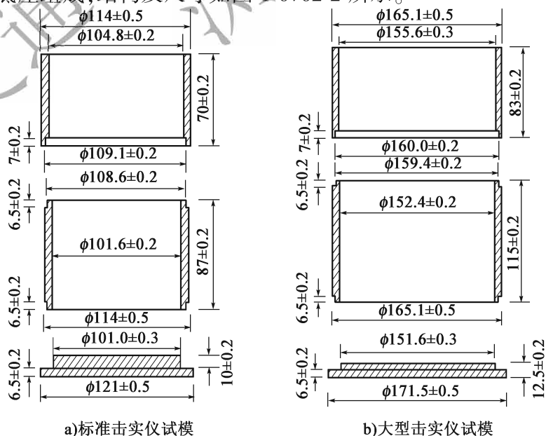
图 T 0702-2 试模 (尺寸单位: mm)
