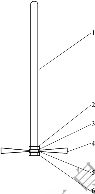
图 T 0658-2 搅拌器 1-搅拌棒;2、6-螺母;3、5-垫圈;4-搅拌叶片
