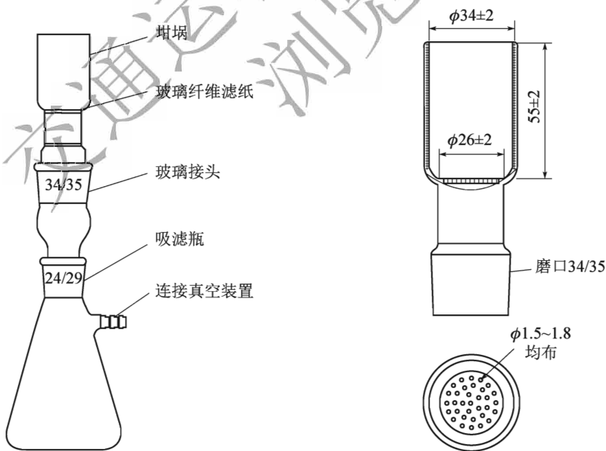
图 T 0607-1 过滤装置
