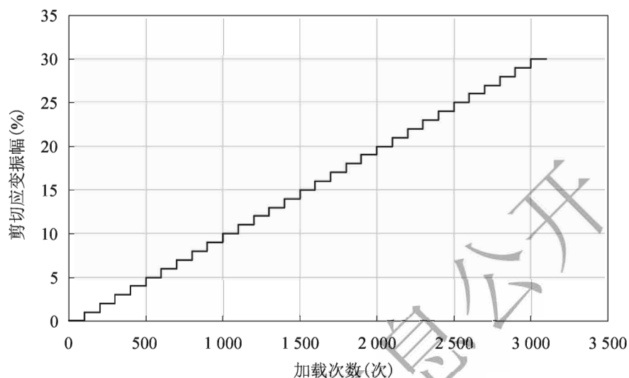
图 T 0648-2 应变扫描试验中应变路径
