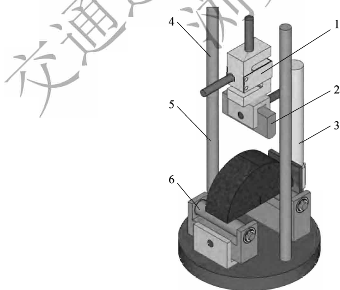
图 T 0744-1 半圆弯曲试验机
