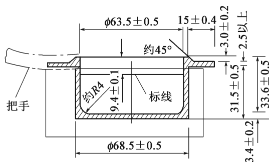
图 T 0611-2 克利夫兰开口杯(尺寸单位:mm)
