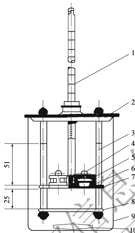
图 T 0606-1 软化点试验仪(尺寸单位:mm)
