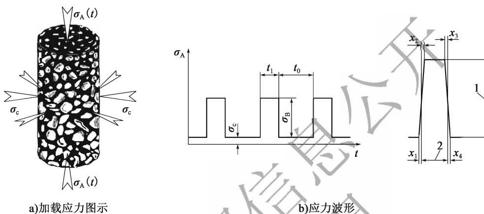
图 T 0745-5 静态围压时三轴加载应力图示和重复加载的轴向应力波形 1-应力强度,2-加载时间
