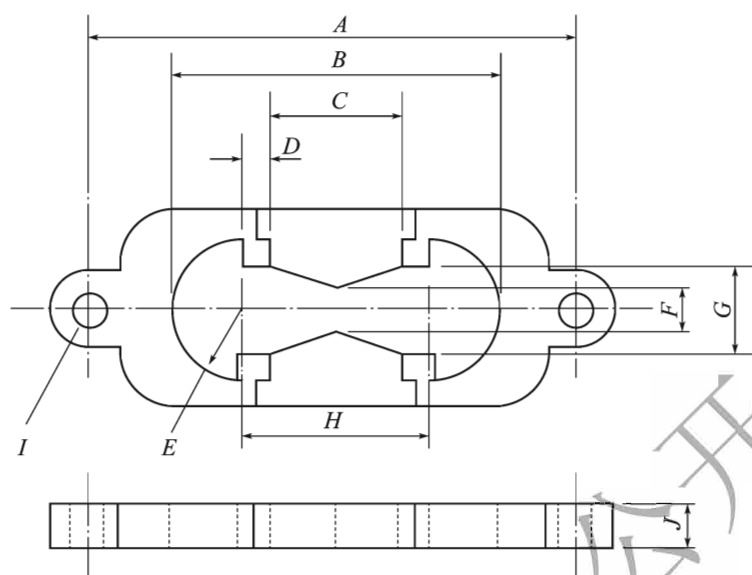
图 T 0605-2 延度仪试模(尺寸单位:mm)
