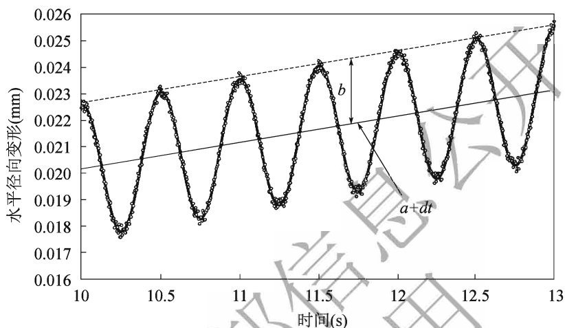
图 T 0743-4 实测的试件水平径向变形-时间曲线
