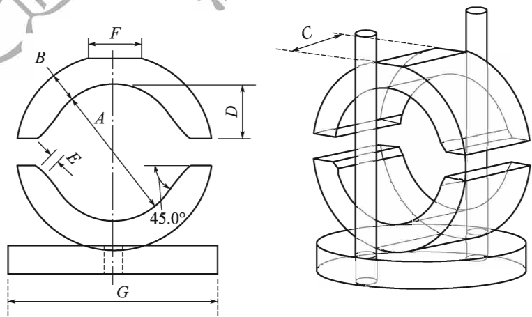
图 T 0709-1 稳定度试验仪压头 (尺寸单位:mm)
