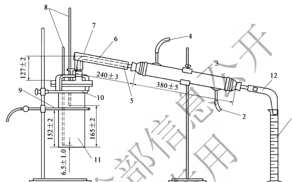
图 T 0667-1 蒸馏装置(尺寸单位:mm)
