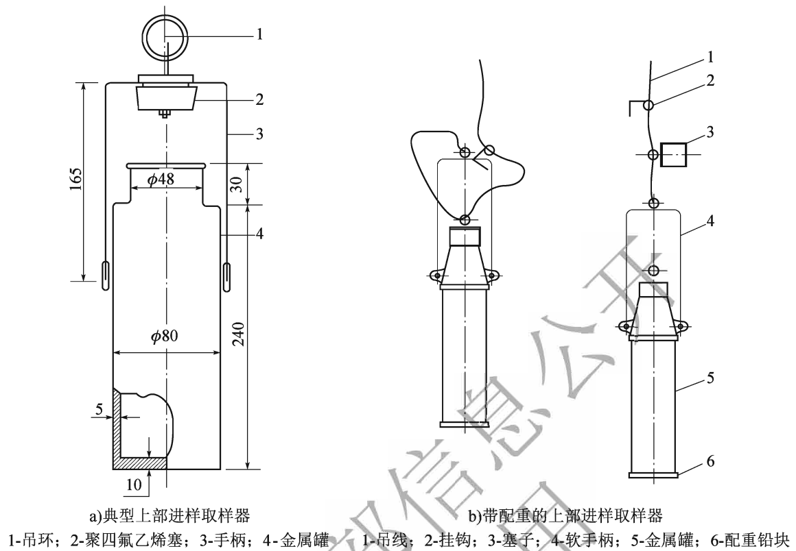
图 T 0601-1 上部进样取样器 (尺寸单位:mm)
