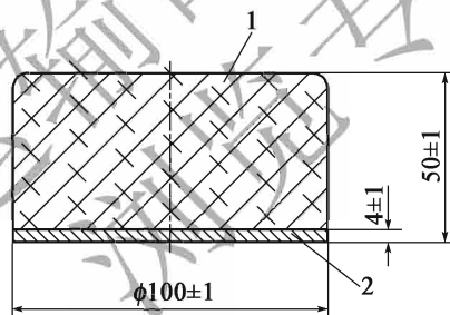
图 T 0763-2 标定块(尺寸单位:mm) 1-橡胶块;2-钢板
