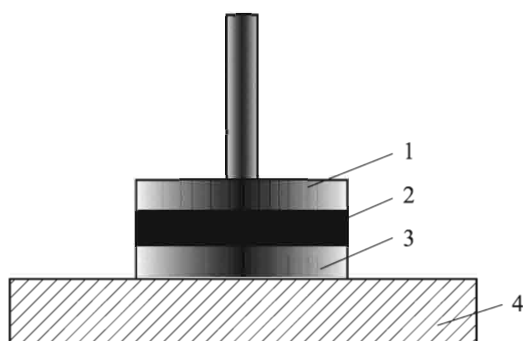
图 T 0628-1 动态剪切流变仪试验盘
