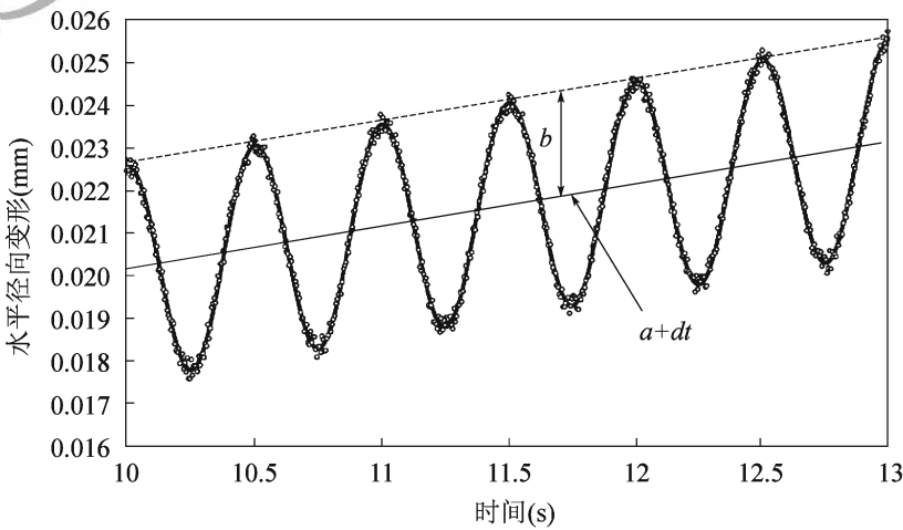
图 T 0742-10 实测的试件水平径向变形-时间曲线
