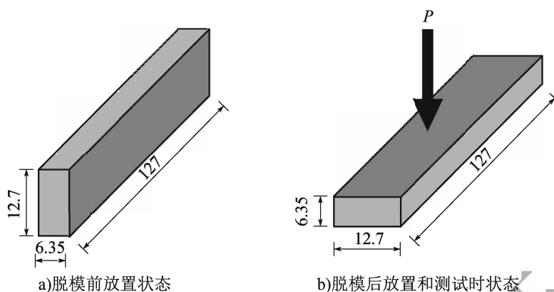
图 T 0627-6 试件脱模前后的状态(尺寸单位:mm)
