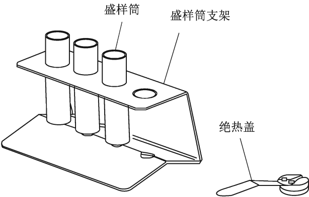
图 T 0625-2 盛样筒支架及绝热盖
