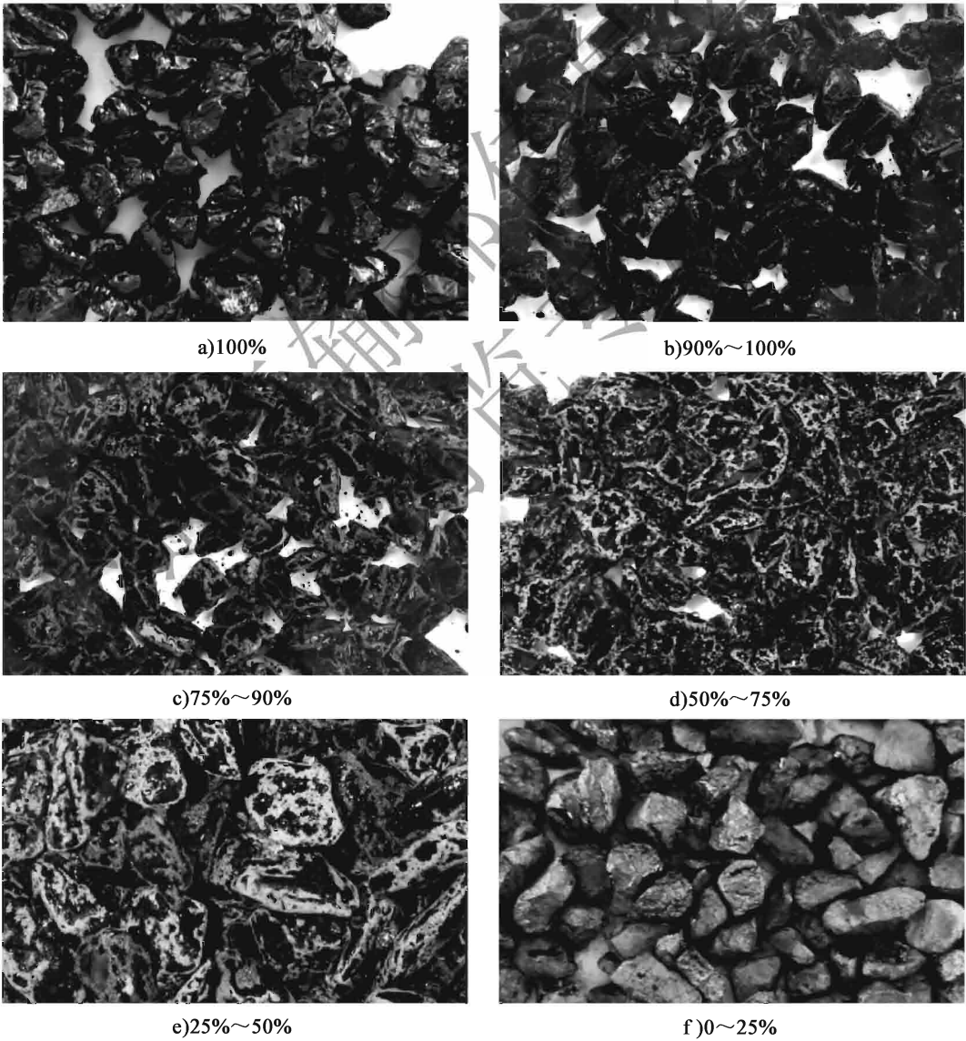
图 T 0616-2 集料不同裹覆率对照情况
