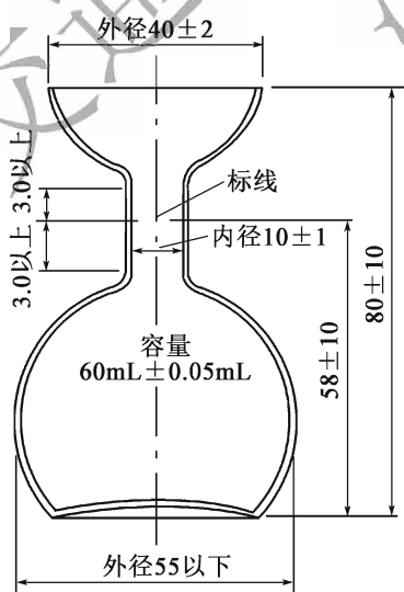
图 T 0623-3 接收瓶(尺寸单位:mm)
