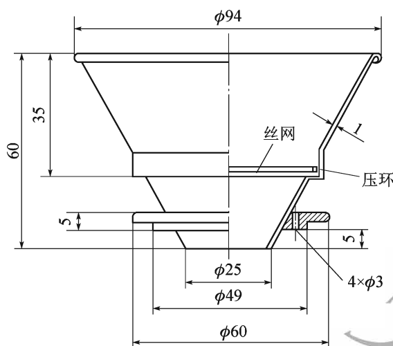
图 T 0602-1 过滤漏斗(尺寸单位:mm)
