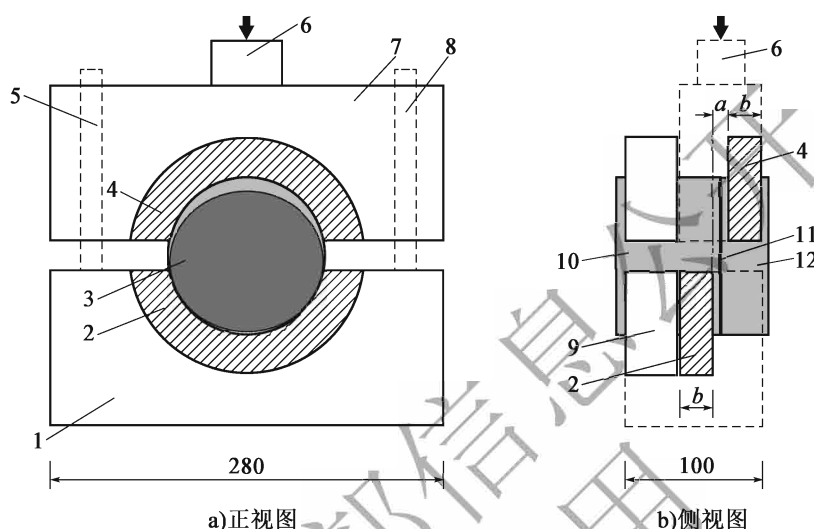
图 T 0772-2 剪切仪剪切图示(尺寸单位:mm)
