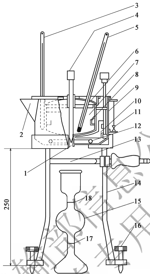
图 T 0622-1 恩格拉黏度计(尺寸单位:mm)
