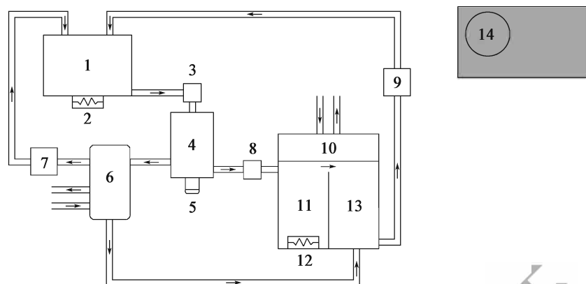
图 T 0722-1 自动抽提仪
