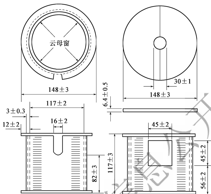
图 T 0632-3 保温罩(尺寸单位:mm)
