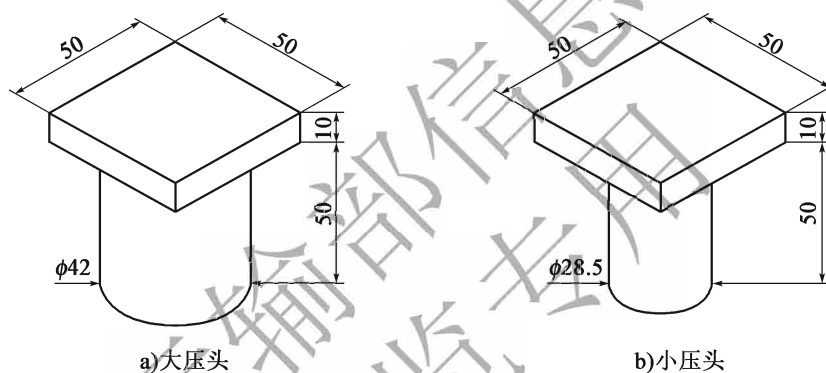
图 T 0746-1 贯入压头(尺寸单位:mm)
