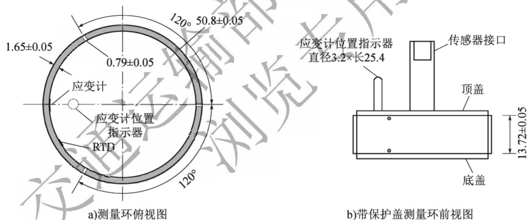
图 T 0649-1 测量环(尺寸单位:mm)
