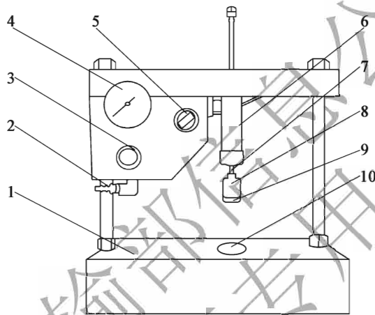
图 T 0754-1 黏聚力试验仪
