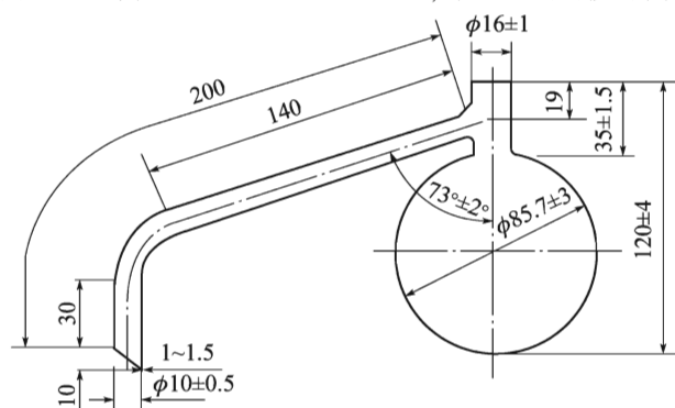
图 T 0615-1 蒸馏烧瓶(尺寸单位:mm)
