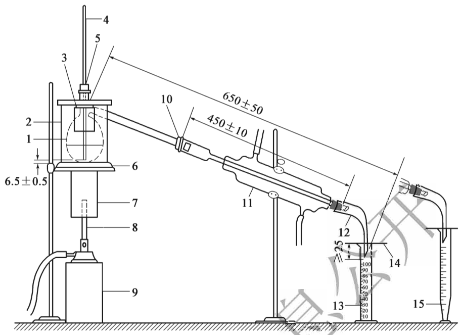
图 T 0632-1 蒸馏装置(尺寸单位:mm)
