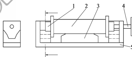
图 T 0748-4 圆柱体试件安装台
