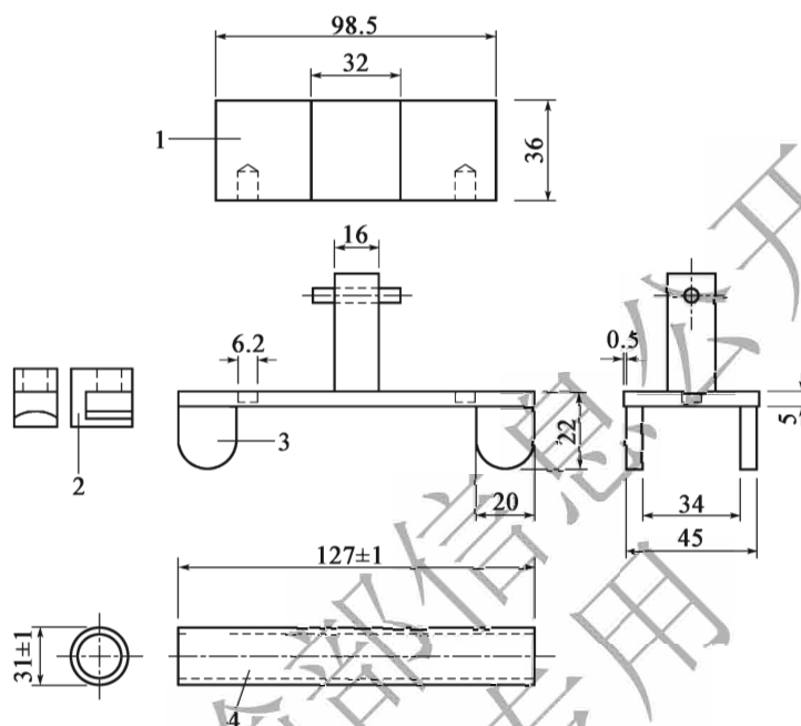
图 T 0752-3 磨耗头(尺寸单位:mm)
