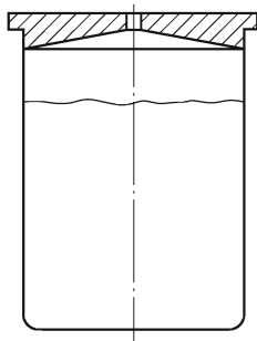
图 T 0603-2 金属比重瓶
