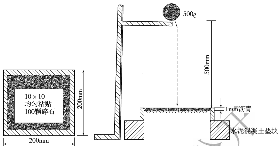
图 T 0660-1 沥青与集料低温黏结性的板冲击试验
