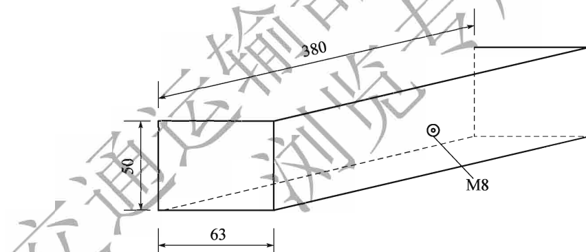
图 T 0739-2 试件长度方向两侧粘贴一个 M8 螺母(尺寸单位:mm)
