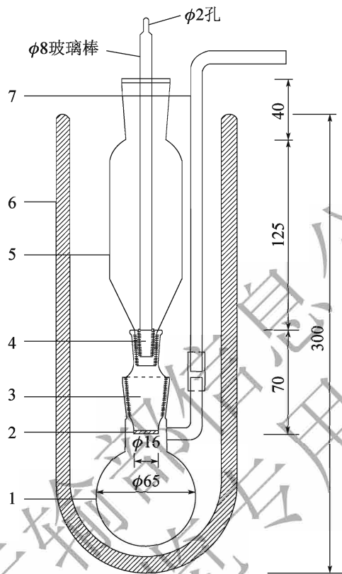
图 T 0615-2 冷却过滤装置 (尺寸单位:mm)
