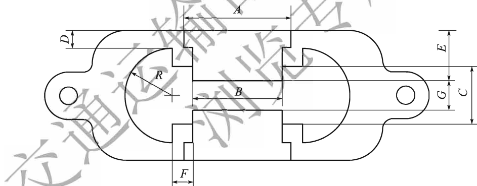
图 T 0662-1 弹性恢复试验用直线延度试模(尺寸单位:mm)
