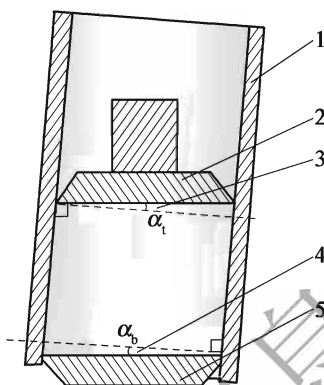
图 T 0736-1 有效内旋转角示意图
