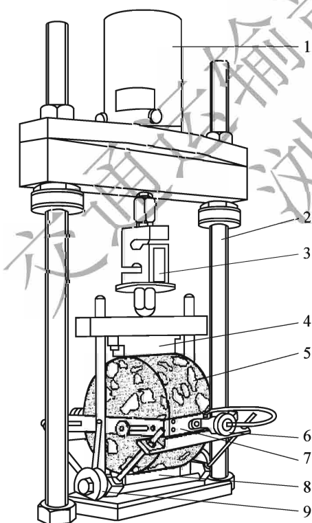
图 T 0742-1 采用 LVDT 传感器的劈裂拉伸动态测试仪 1-动力制动器;2-钢制加载架;3-荷载传感器;4-上压条;5-试件; 6-位移传感器调节器;7-位移传感器安装框架;8-下压条;9-位 移传感器对夹具
