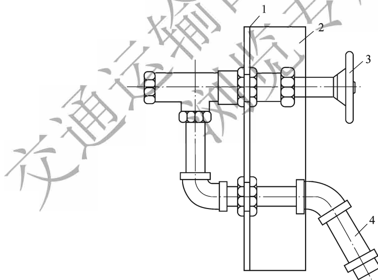
图 T 0601-4 罐壁上的取样阀 1-罐壁;2-保温层;3-阀门;4-放样口
