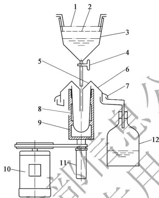
图 T 0722-6 连续流式离心机结构示意图
