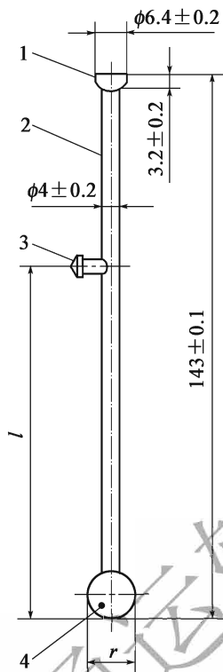
图 T 0621-3 球塞 (尺寸单位:mm) 1-半球形顶部;2-杆;3-水平挂钉;4-球
