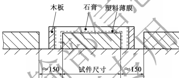
图 T 0701-2 切割取样示意图(尺寸单位:mm)
