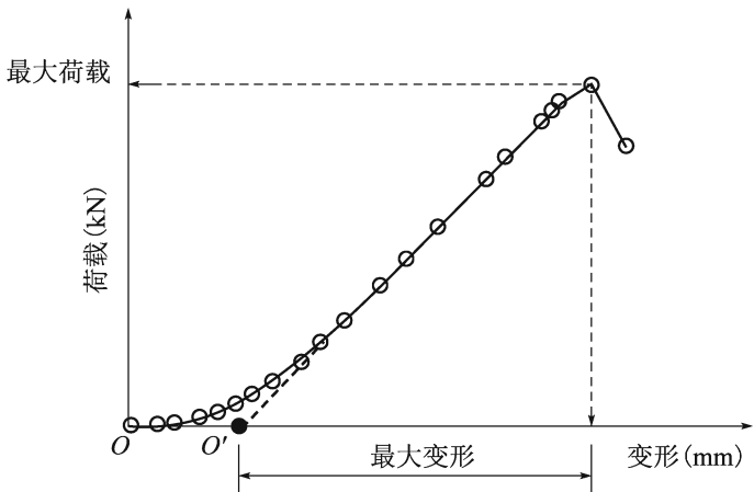
图 T 0716-4 劈裂试验的荷载-变形曲线
