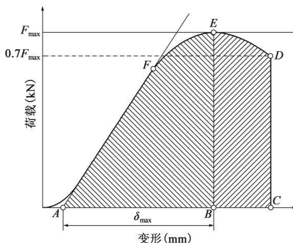
图 T 0772-5 直接剪切试验位移-荷载曲线
