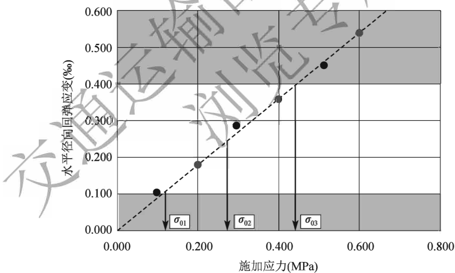
图 T 0743-2 根据应力-水平径向回弹应变曲线确定施加应力水平
