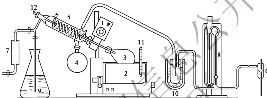
图 T 0727-1 旋转蒸发器沥青回收装置(加气式)
