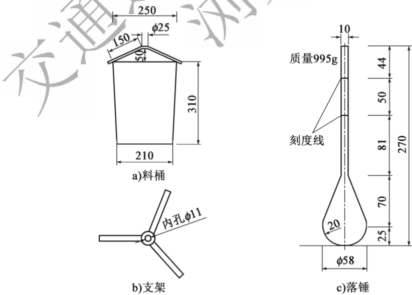
图 T 0764-1 流动性试验仪(尺寸单位:mm)
