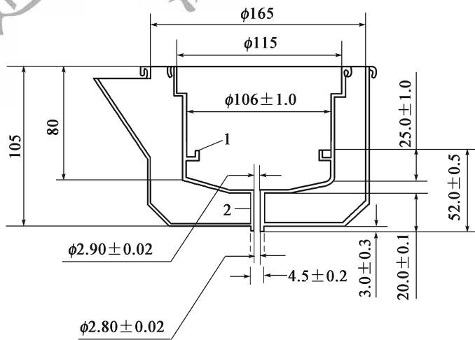
图 T 0622-2 黏度杯(尺寸单位:mm)
