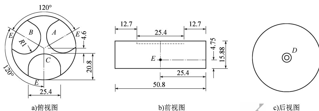
图 T 0627-4 高度量块(尺寸单位:mm)
