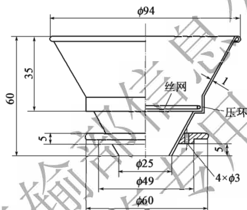
图 T 0621-5 过滤漏斗(尺寸单位:mm)
