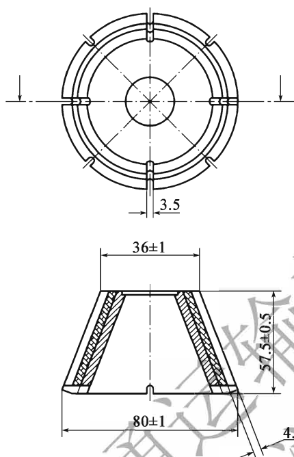
图 T 0760-3 磨光滚轮(尺寸单位:mm)
