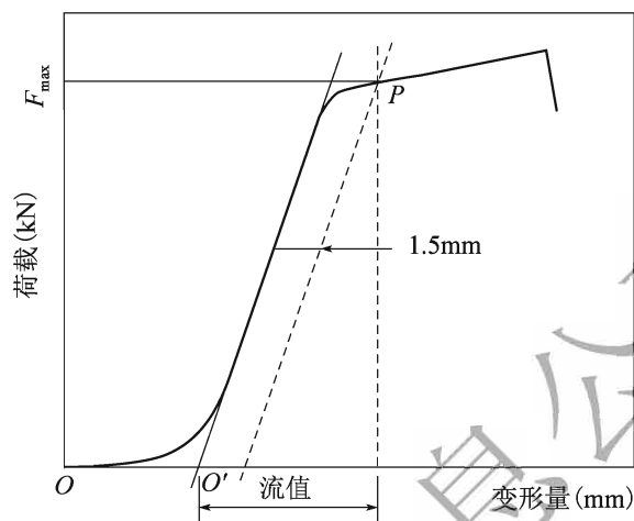
图 T 0709-3 稳定度-变形量曲线无峰值的修正示意图
