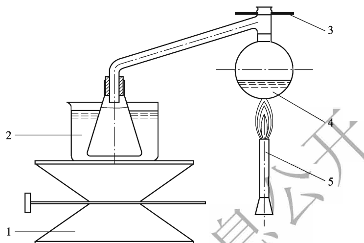
图 T 0615-4 蒸馏装置
