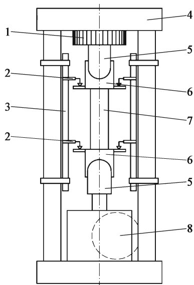
图 T 0748-1 位移传感器内置式低温约束应力试验仪 1-荷载传感器;2-位移传感器;3-温差测量基座;4-加载架;5-万向接头;6-连接器;7-试件;8-带步进电机的齿轮箱
