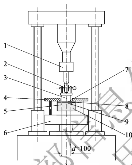
图 T 0773-1 拉伸仪(尺寸单位:mm)
