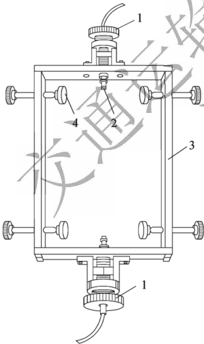
图 T 0742-3 水平径向位移测量系统 1-LVDT 调节螺栓;2-LVDT 位移传感器;3-LVDT 安装框架;4-固定夹具
