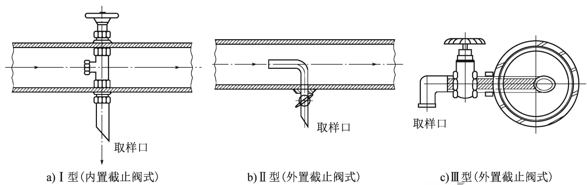
图 T 0601-5 管线上的取样管
