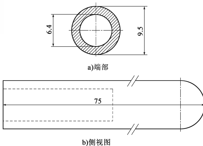
图 T 0768-2 贯入杆(尺寸单位:mm)
