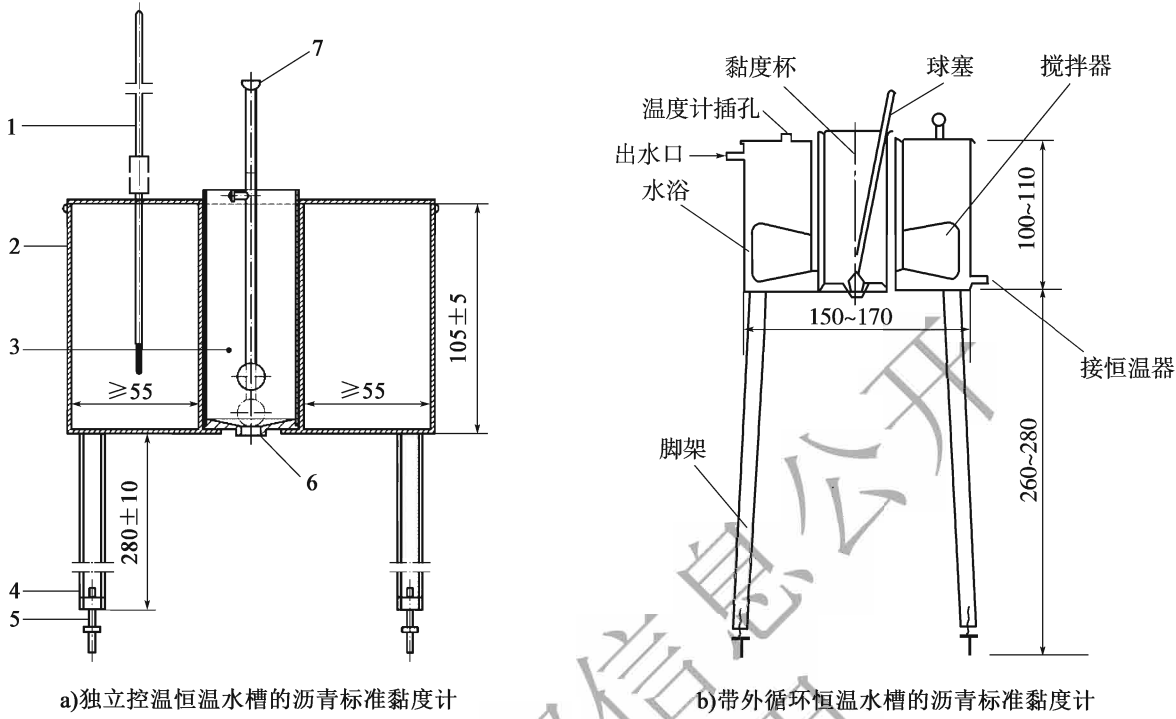
图 T 0621-1 沥青标准黏度计(尺寸单位:mm)
