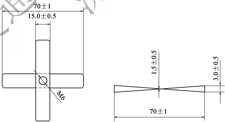
图 T 0658-4 搅拌叶片(尺寸单位:mm)
