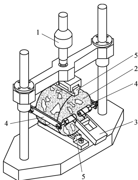
图 T 0742-2 采用引伸计的劈裂拉伸动态测试仪 1-动力制动器;2-试件;3-引伸计;4-变形条;5-上、 下压条
