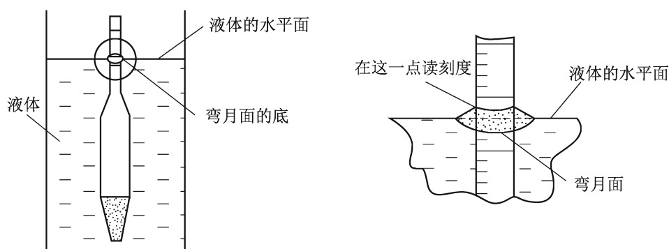
图 T 0603-3 密度计试验读数示意图
