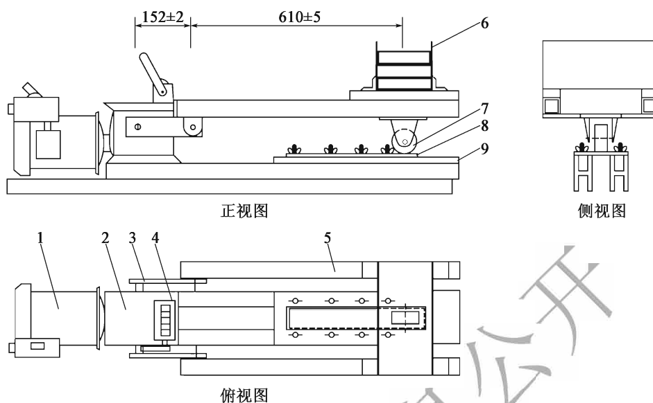
图 T 0755-1 负荷轮测试仪(尺寸单位:mm)
