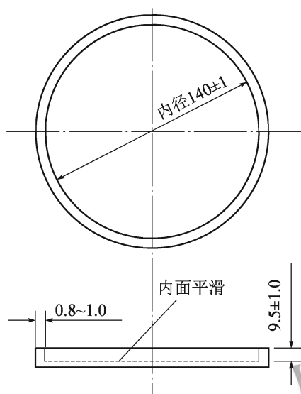
图 T 0609-3 盛样盘 (尺寸单位:mm)
