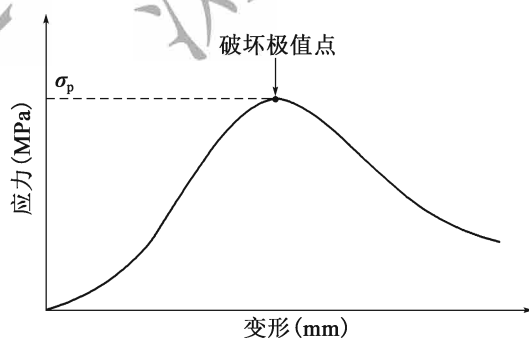
图 T 0746-2 单轴贯入试验典型应力-变形曲线
