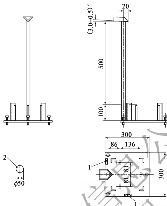
图 T 0771-2 三点支架(尺寸单位:mm)
