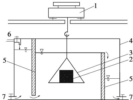
图 T 0705-1 溢流水箱及下挂法水中重称量方法示意图
