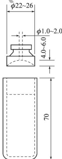
图 T 0603-1 玻璃比重瓶(尺寸单位:mm)
