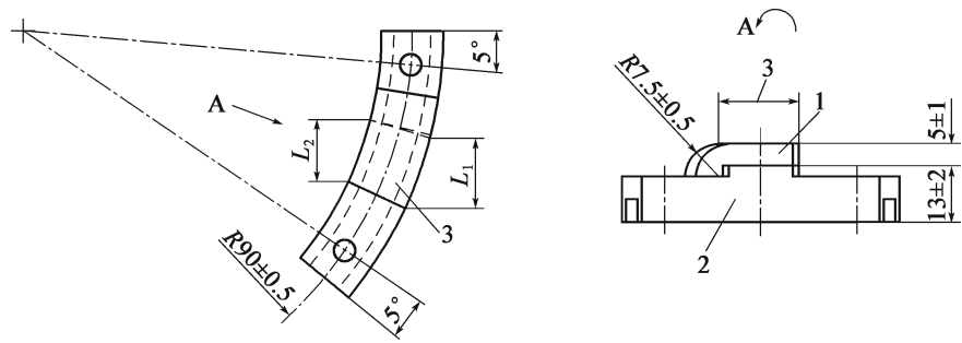
图 T 0760-6 滑块(尺寸单位:mm) 1-橡胶片;2-金属底座;3-平均接触长度 注: L_1 和 L_2 的平均值为 30\text{mm} \pm 1\text{mm} 。
