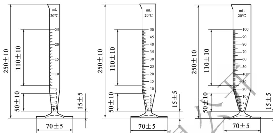
图 T 0632-4 下异径量筒(尺寸单位:mm)
