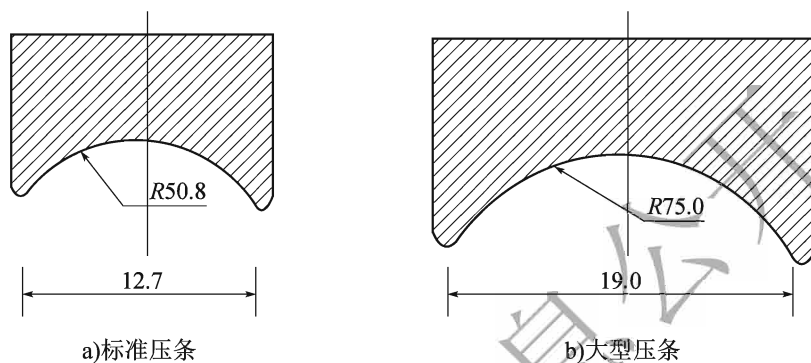
图 T 0742-5 压条(尺寸单位:mm)
