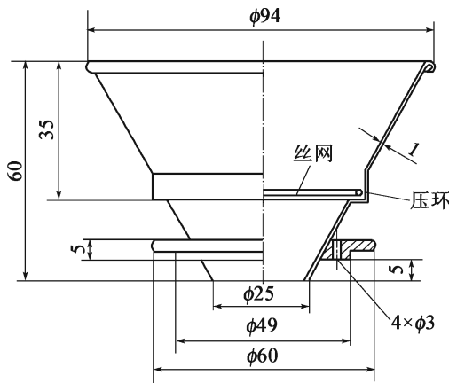
图 T 0622-4 过滤漏斗 (尺寸单位:mm)
