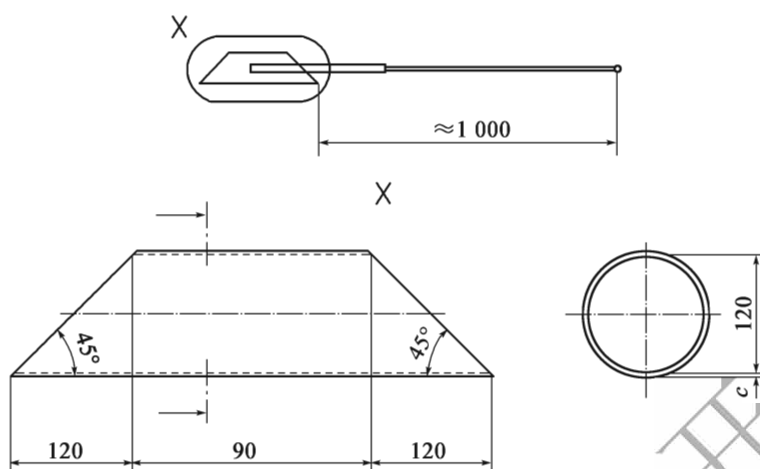
图 T 0701-1 取样管(尺寸单位:mm)
