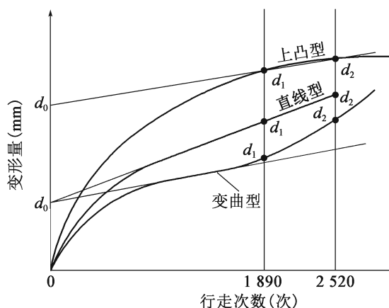
图 T 0719-2 车辙变形量-行走次数曲线
