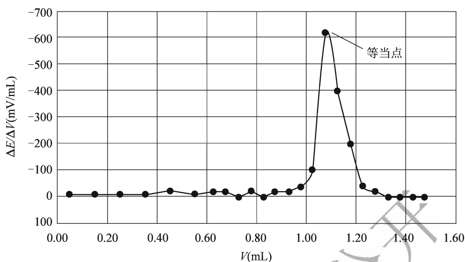
图 T 0626-1 电位滴定试验 \Delta E/\Delta V - V 曲线示例
