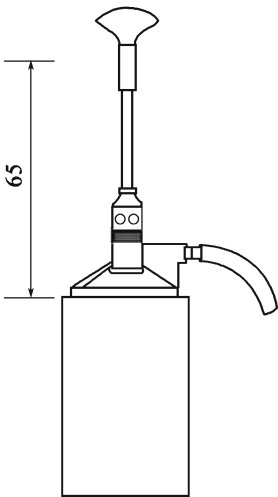
图 T 0667-5 扇形燃气灯(尺寸单位:mm)
