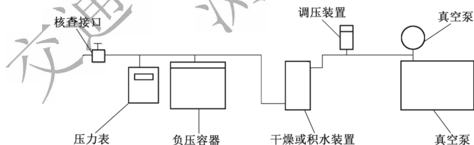
图 T 0711-1 真空负压装置
