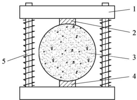
图 T 0716-1 劈裂试验加载方式示意图 1-上压头;2-上压条;3-试件;4-下压条;5-导杆
