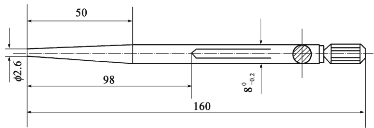
图 T 0622-3 硬木塞 (尺寸单位:mm)
