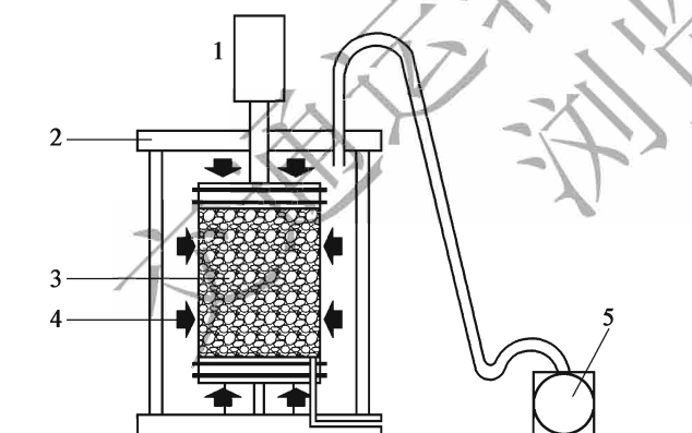
图 T 0745-1 A 型三轴重复压缩试验装置 1-动力制动器;2-压力室;3-试件;4-围压;5-真空泵
