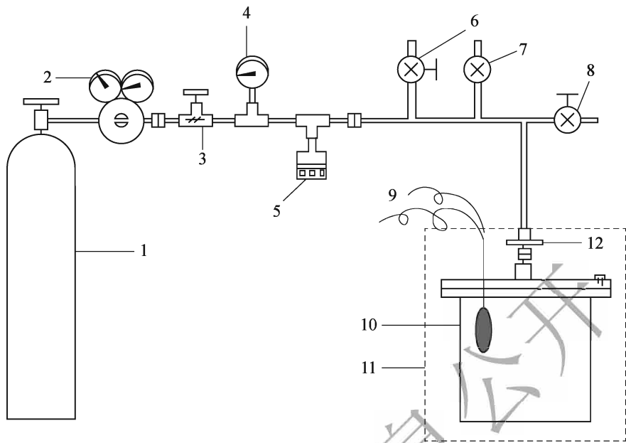
图 T 0630-1 压力老化试验仪 (PAV)
