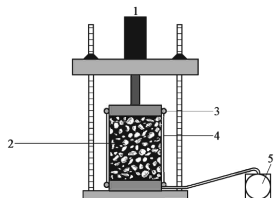
图 T 0745-3 C 型三轴重复压缩试验装置 1-动力制动器;2-试件;3-O 形环;4-真空膜;5-真空泵
