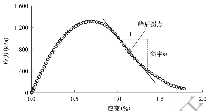
图 T 0765-1 劈裂试验的应力-变形曲线
