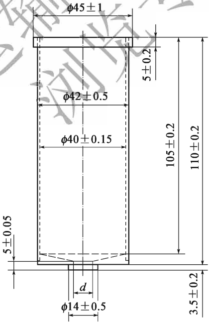
图 T 0621-2 黏度杯(尺寸单位:mm)
