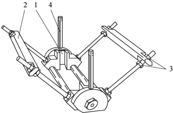
图 T 0742-4 LVDT 对中夹具 1-加载框架的定位槽;2-LVDT 对中框架;3-对中条调节螺栓;4-对中条释放杆
