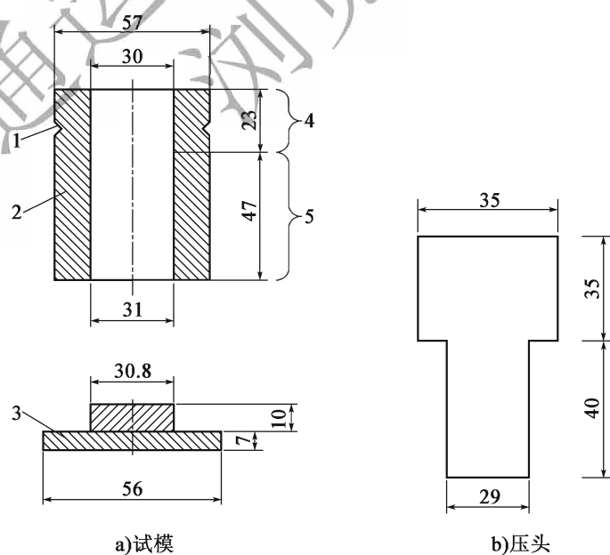
图 T 0758-3 试模(尺寸单位:mm)
